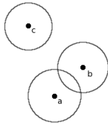
Figure 1: Aura-nimbus IM
