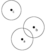
Figure 1: Aura-nimbus IM
