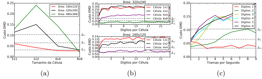
Figura 5: Impacto da escolha de parâmetros na observabilidade dos fluxos.
