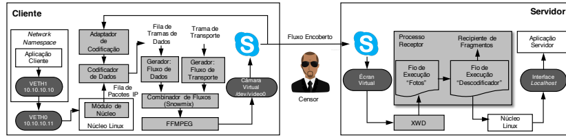
Figura 1: Componentes do protótipo (caixas sombreadas).
