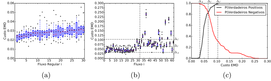
Figura 4: Custo EMD como classificador de fluxos Skype.
