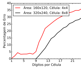
Figura 6: Taxa de erros.
